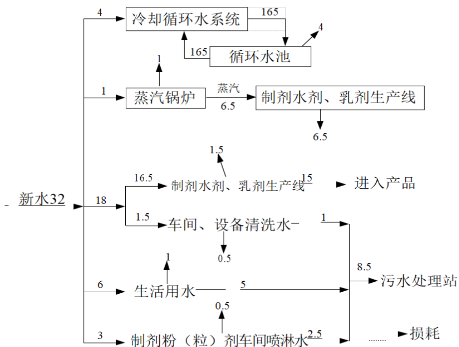
图 3-1 水平衡图 (m 3 /d)
