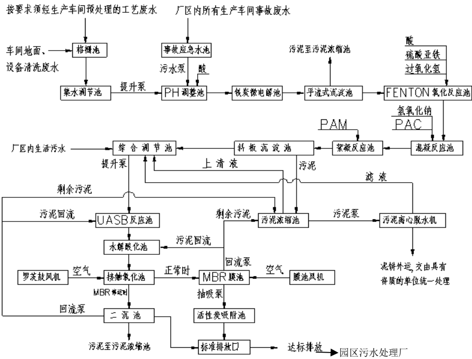
图4-1 废水治理流程示意图
