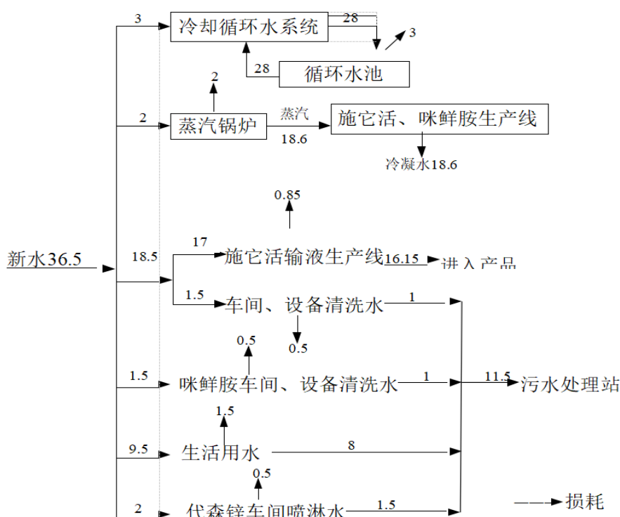
图 3-1 水平衡图 (m 3 /d)
