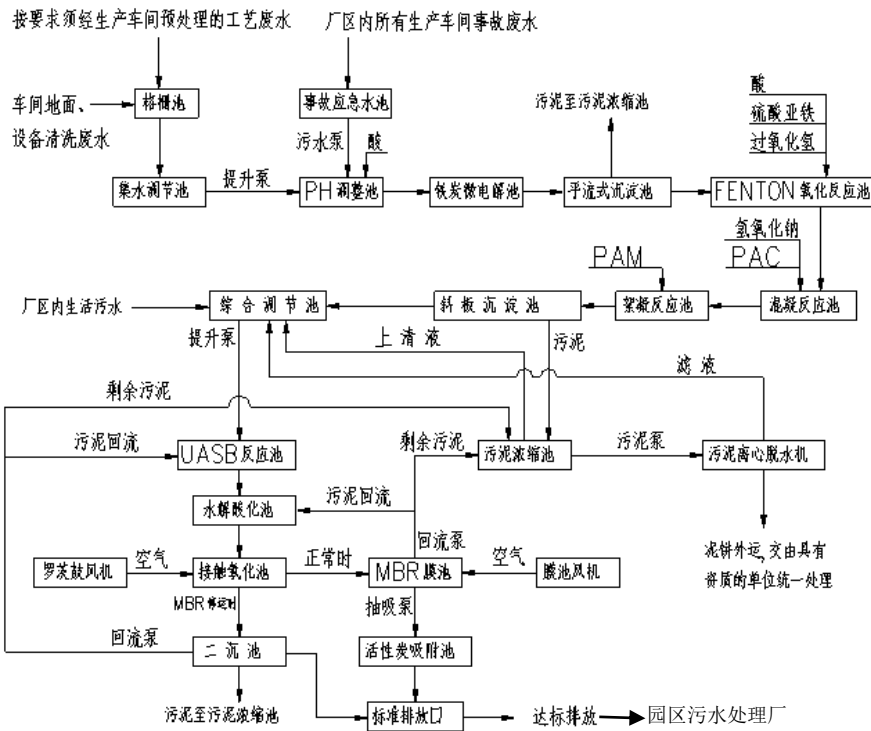
图4-1 废水治理流程示意图
